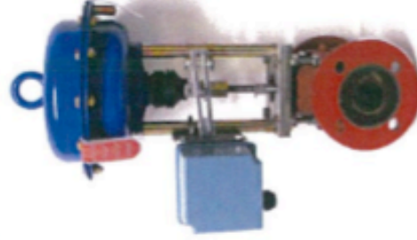
VALVOLA PNEUMATICA A MEMBRANA MODELLO S+S ATTUATORE PNEUMATICO A SEPLICE EFFETTO CONTATTI DI FINECORSA ECKARDT SGE985
