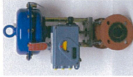
VALVOLA PNEUMATICA A MEMBRANA MODELLO S+S ATTUATORE PNEUMATICO A SEPLICE EFFETTO POSIZIONATORE PNEUMATICO ECKARDT SRI990-B
