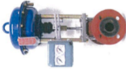
VALVOLA PNEUMATICA A MEMBRANA MODELLO S+S ATTUATORE PNEUMATICO A SEPLICE EFFETTO POSIZIONATORE PNEUMATICO ECKARDT SRP981-B
