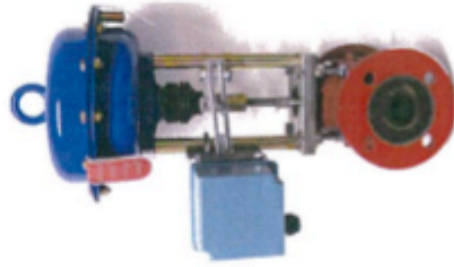
VALVOLA PNEUMATICA A MEMBRANA MODELLO S+S ATTUATORE PNEUMATICO A SEPLICE EFFETTO POSIZIONATORE ELETTRO-PNEUMATICO ECKARDT SRI986-B
